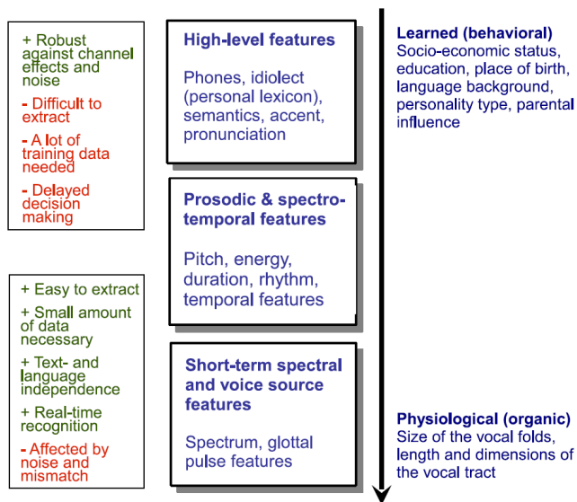
Figure 4: 基于知识驱动的特征设计 [3]
