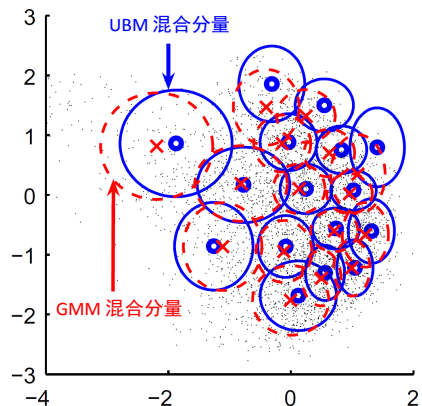
Figure 5: 基于MAP的GMM-UBM模型 [5]
