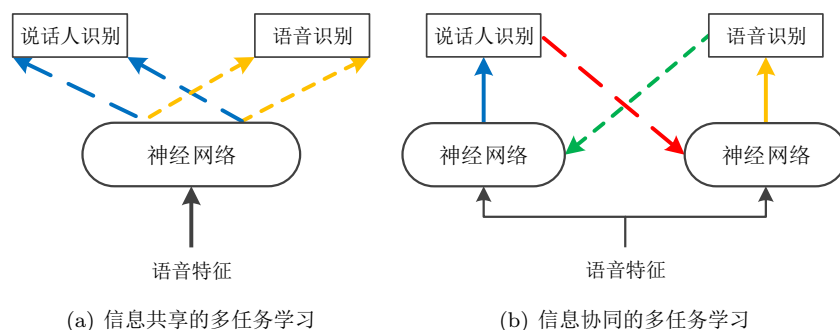
Figure 10: 两种多任务学习的模型结构
