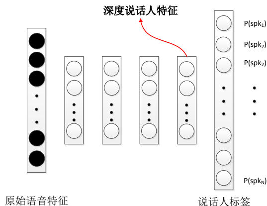
Figure 9: 基于DNN 的说话特征学习
