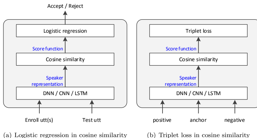
Figure 11: 两种“端到端”的识别模型
